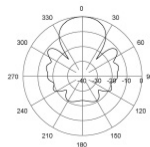
H-Plane | 385 MHz
