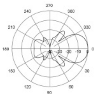
E-Plane | 385 MHz
