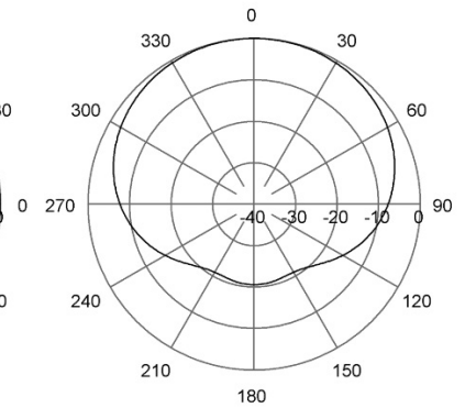
H-Plane | 147 MHz
